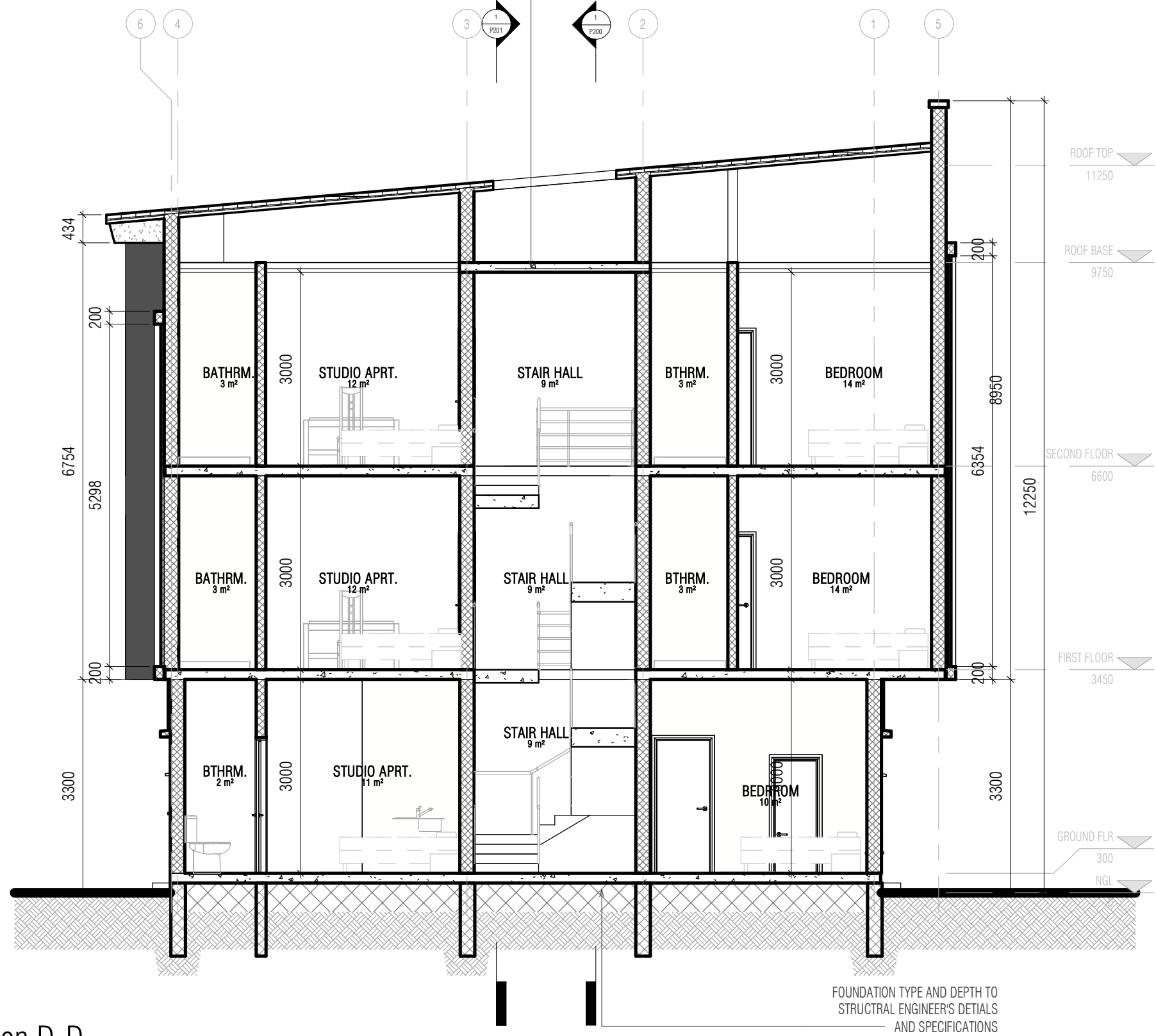
1 Section D-D 1 : 75
